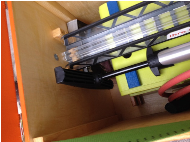
Pumpengriff neben Leiter positionieren
